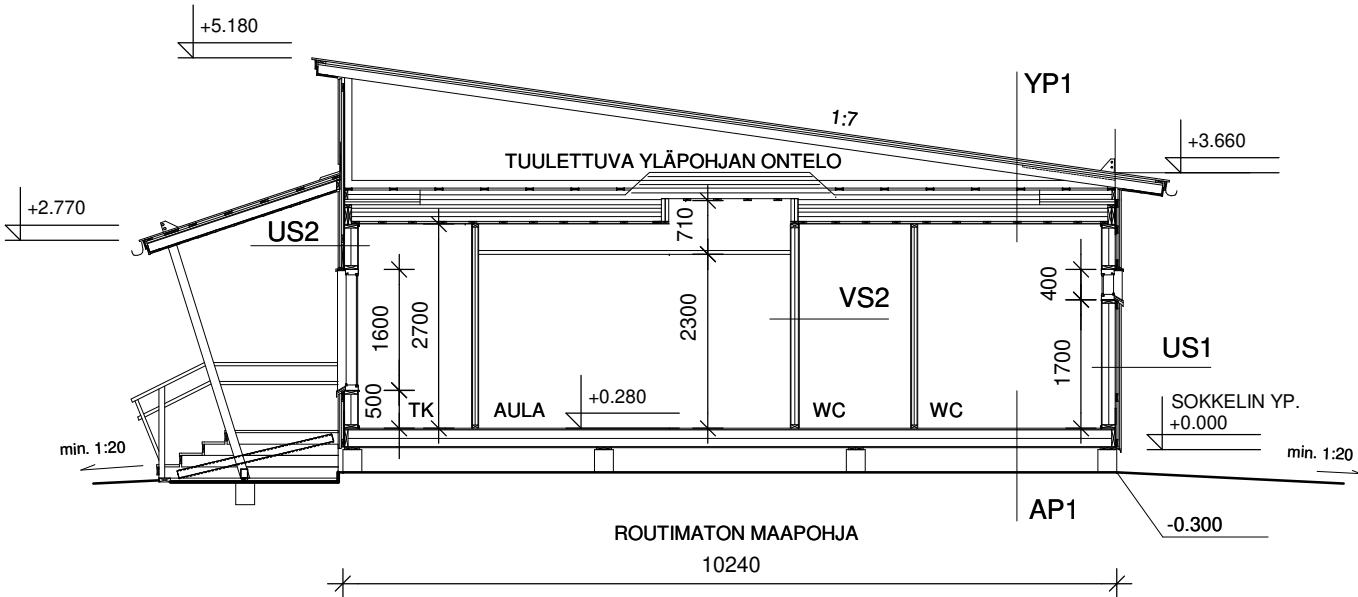
LEIKKAUS A - A
