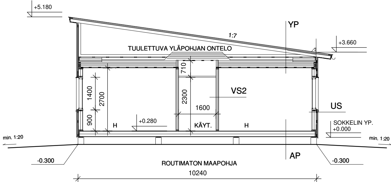
LEIKKAUS B - B
